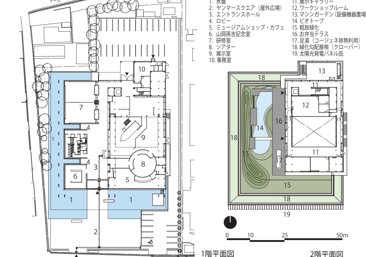
□1階平面図 □2階平面図 1:1000
